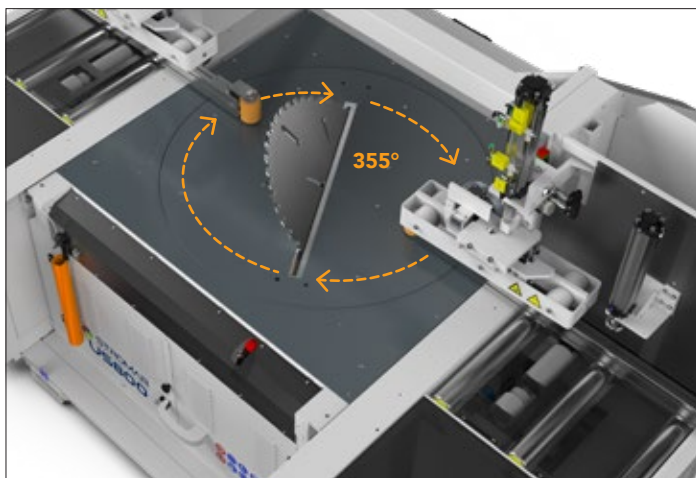
Rotazione piano: 0° ÷ 355°.
