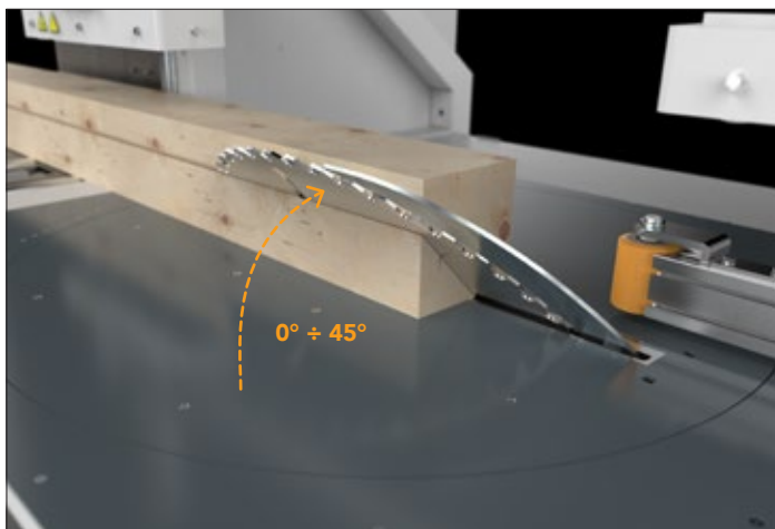
Inclinazione lama: 0° ÷ 45°.
